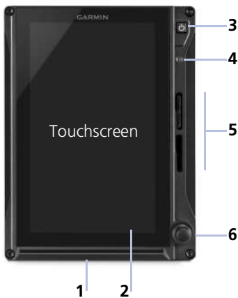
GDU 700P
