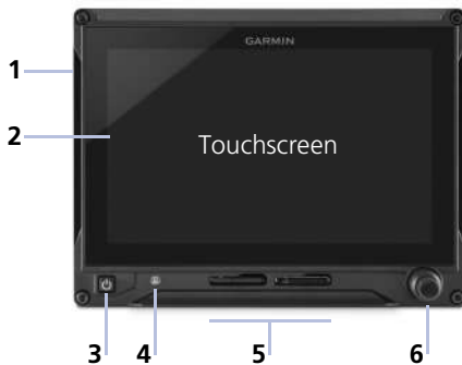
GDU 700L
